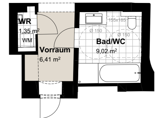
VARIANTE BARRIEREFREIE SANITÄRRÄUME M 1:100
