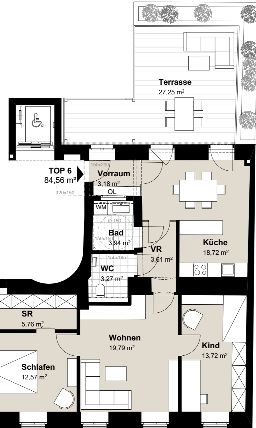
WOHNUNGSPLAN M 1:100
