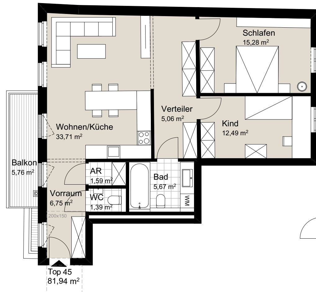
VARIANTE BARRIEREFREIE SANITÄRRÄUME M 1:100
