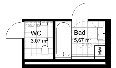
VARIANTE BARRIEREFREIE SANITÄRRÄUME M 1:100
