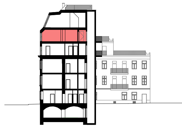
SCHNITT M 1:500
