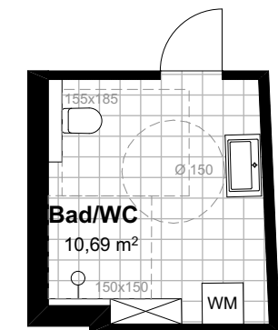
VARIANTE BARRIEREFREIE SANITÄRRÄUME M 1:100
