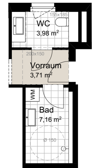
VARIANTE BARRIEREFREIE SANITÄRRÄUME M 1:100
