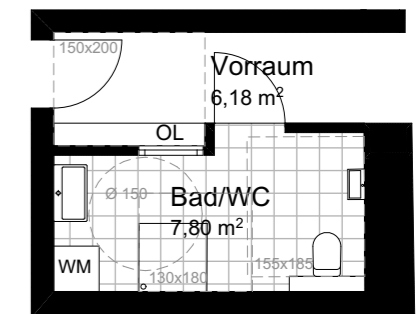
VARIANTE BARRIEREFREIE SANITÄRRÄUME M 1:100
