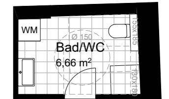
VARIANTE BARRIEREFREIE SANITÄRRÄUME M 1:100
