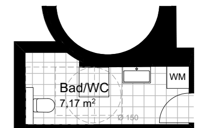
VARIANTE BARRIEREFREIE SANITÄRRÄUME M 1:100
