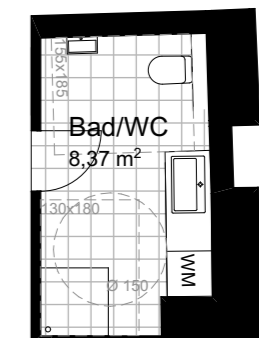
VARIANTE BARRIEREFREIE SANITÄRRÄUME M 1:100
