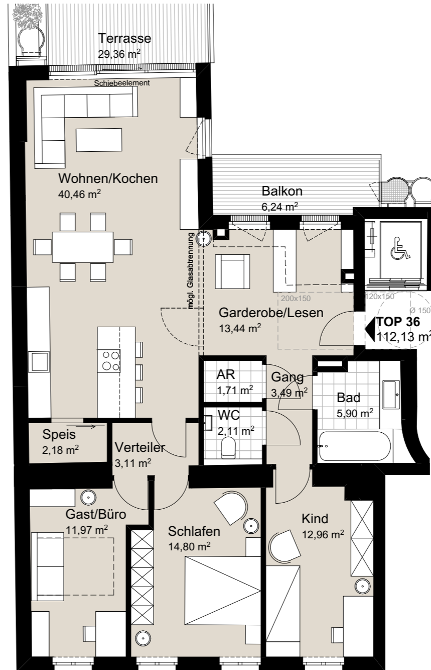
WOHNUNGSPLAN M 1:100
