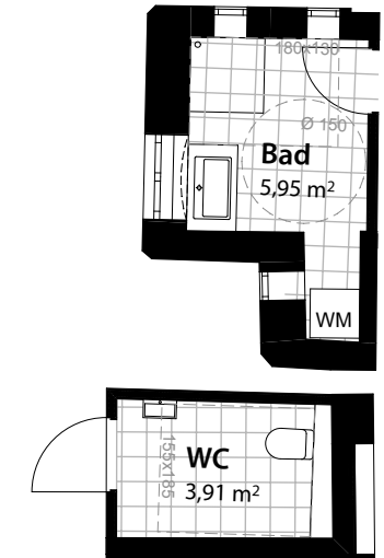
VARIANTE BARRIEREFREIE SANITÄRRÄUME M 1:100
