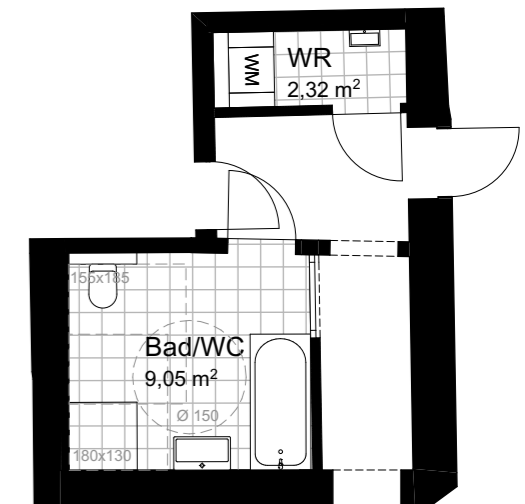
VARIANTE BARRIEREFREIE SANITÄRRÄUME M 1:100
