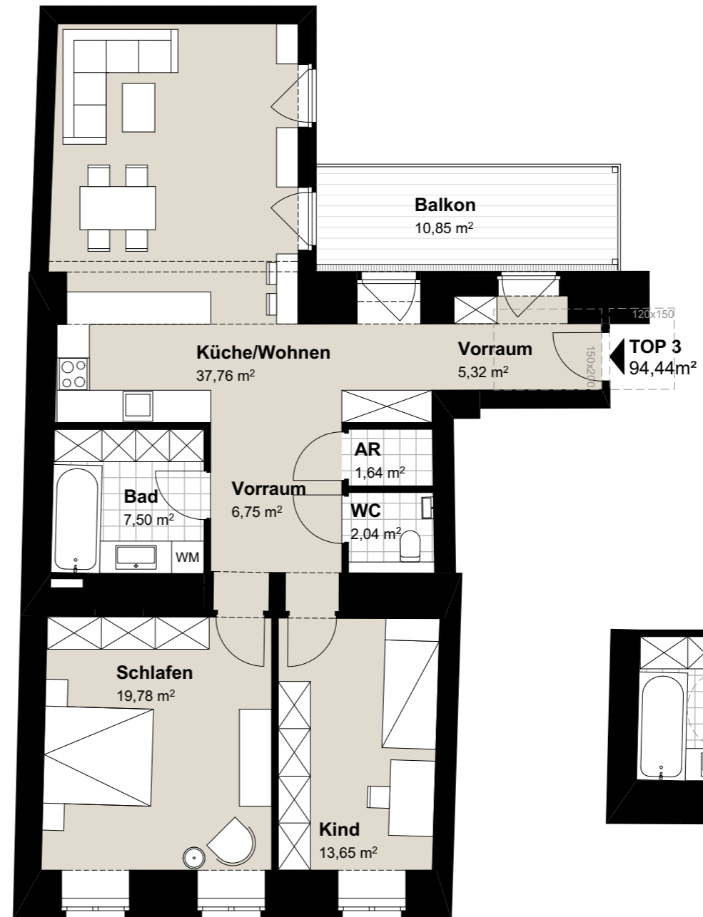
WOHNUNGSPLAN M 1:100
