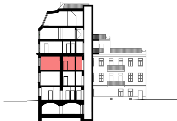
SCHNITT M 1:500
