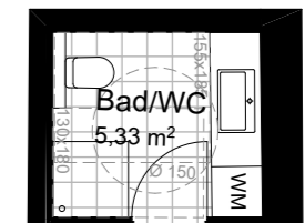
VARIANTE BARRIEREFREIE SANITÄRRÄUME M 1:100
