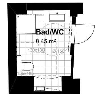
VARIANTE BARRIEREFREIE SANITÄRRÄUME M 1:100
