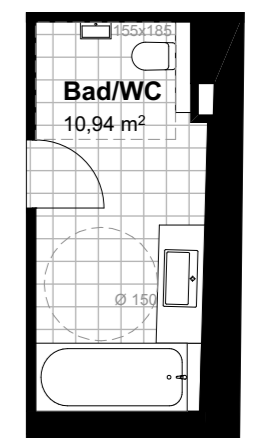
VARIANTE BARRIEREFREIE SANITÄRRÄUME M 1:100
