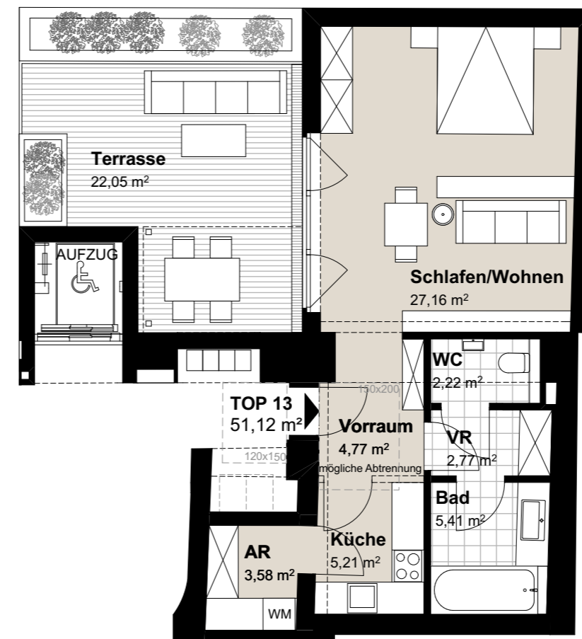
WOHNUNGSPLAN M 1:100
