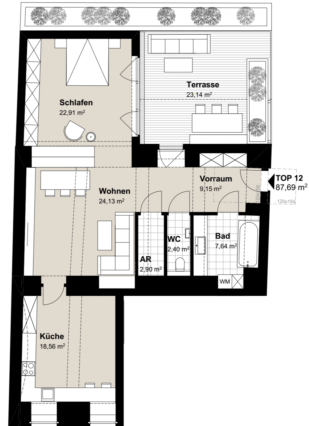
WOHNUNGSPLAN M 1:100
