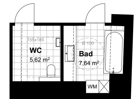
VARIANTE BARRIEREFREIE SANITÄRRÄUME M 1:100
