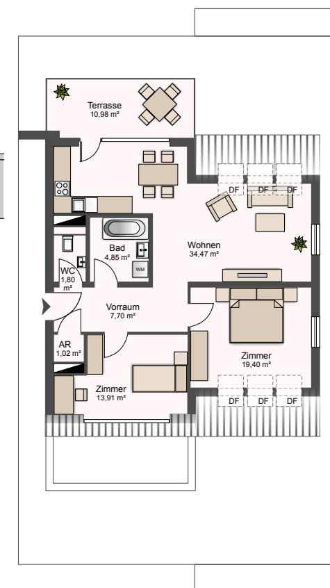
WOHNUNGSGRUNDRISS
