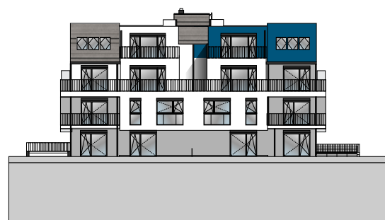
ANSICHT NORD
