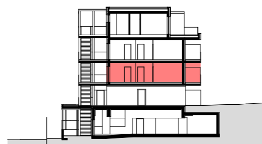
SCHNITT M 1:500
