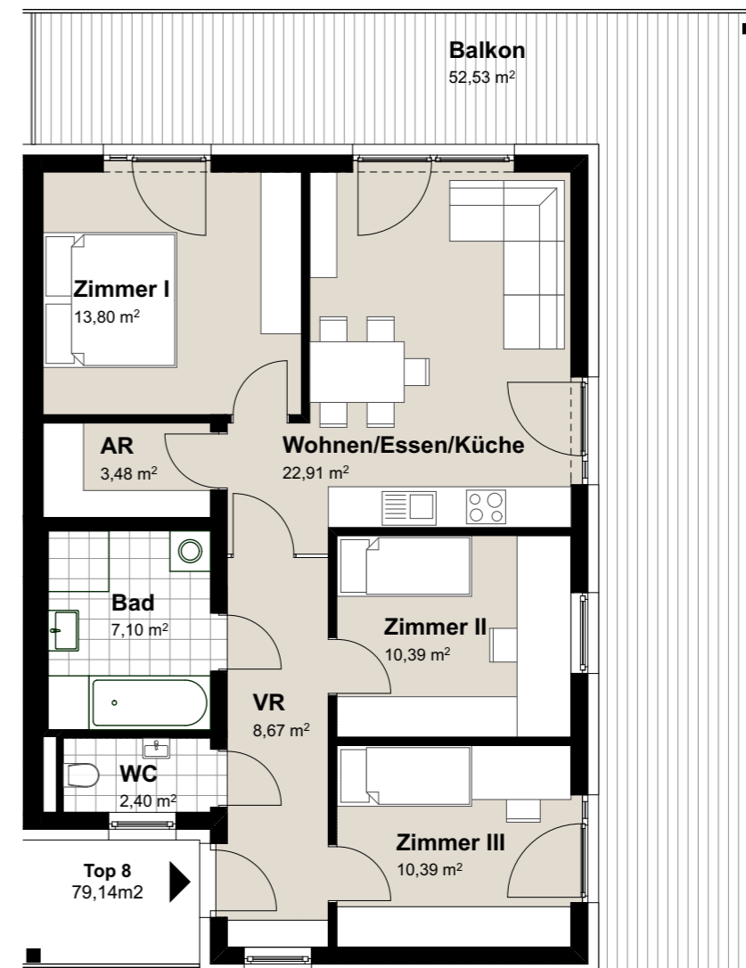
WOHNUNGSPLAN M 1:100
