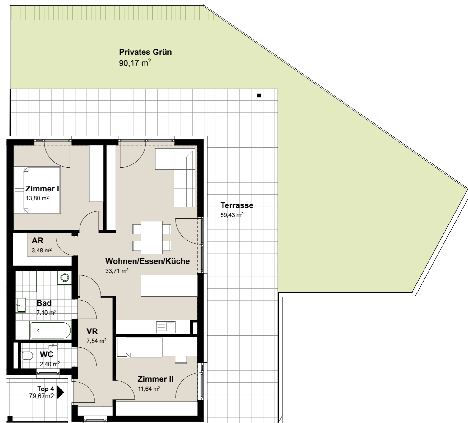
WOHNUNGSPLAN M 1:100
