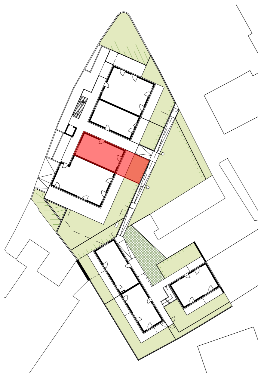
ÜBERSICHTSPLAN EG M 1:500
