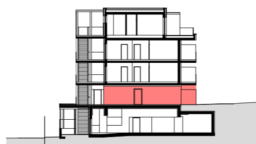
SCHNITT M 1:500
