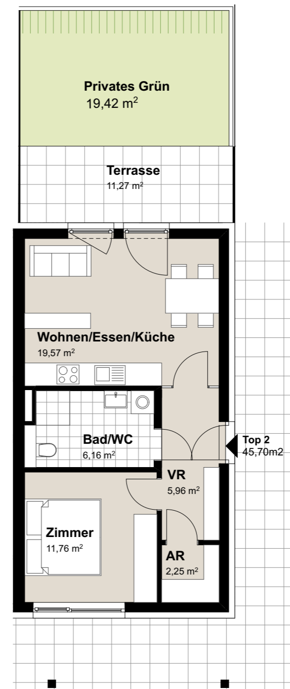
WOHNUNGSPLAN M 1:100
