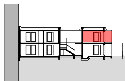
SCHNITT M 1:500
