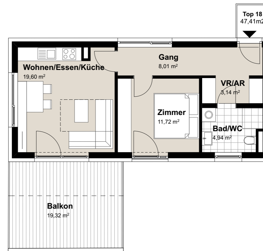
WOHNUNGSPLAN M 1:100
