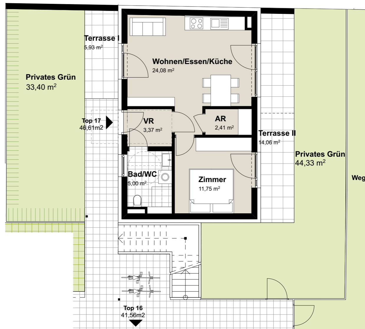
WOHNUNGSPLAN M 1:100
