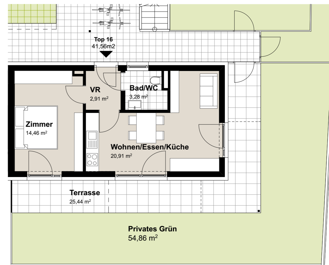
WOHNUNGSPLAN M 1:100
