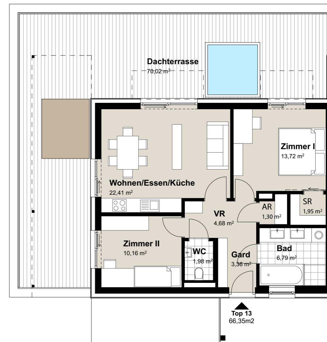
WOHNUNGSPLAN M 1:100
