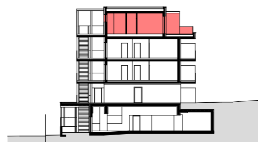
SCHNITT M 1:500
