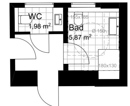
VARIANTE BARRIEREFREIE SANITÄRRÄUME M 1:100
