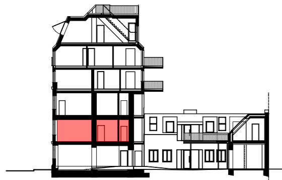
SCHNITT M 1:500
